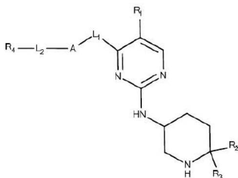
fórmula I
